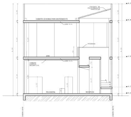
CORTE A-A ESC. 1/50
